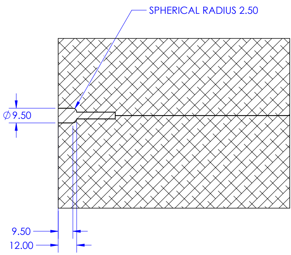
SECTION A-A SCALE 2 : 3
